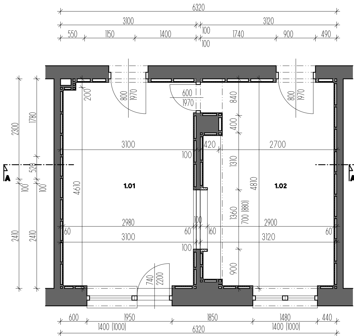
PÔDORYS IZBY - EXISTUJÚCI STAV M 1:50
