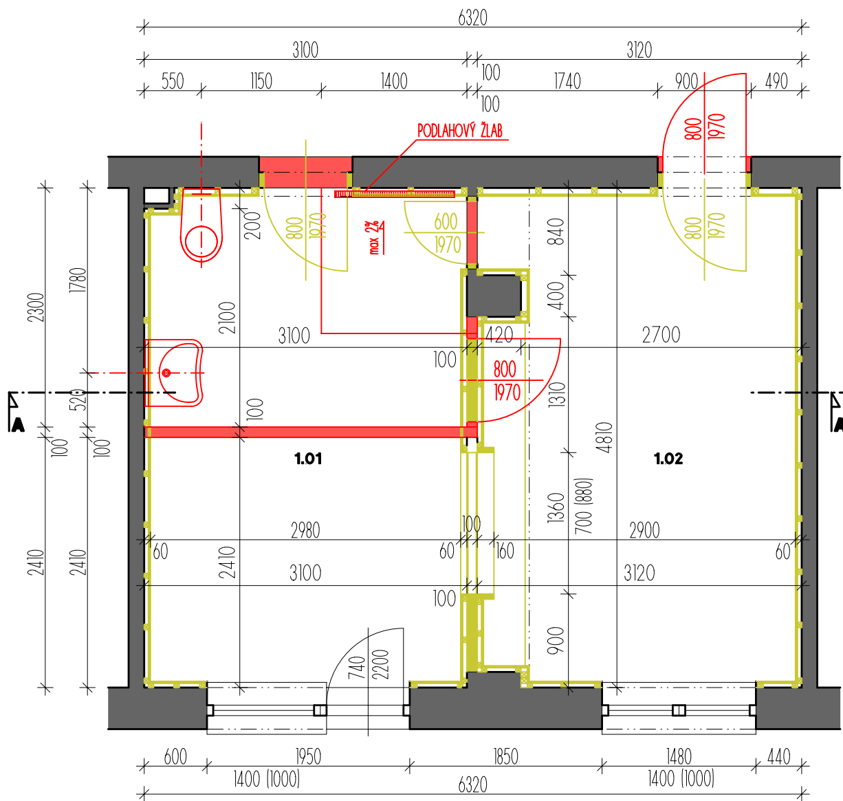
PŮDORYS IZBY - BŮRACIE A MUROVACIE PRÁCE M 1:50
