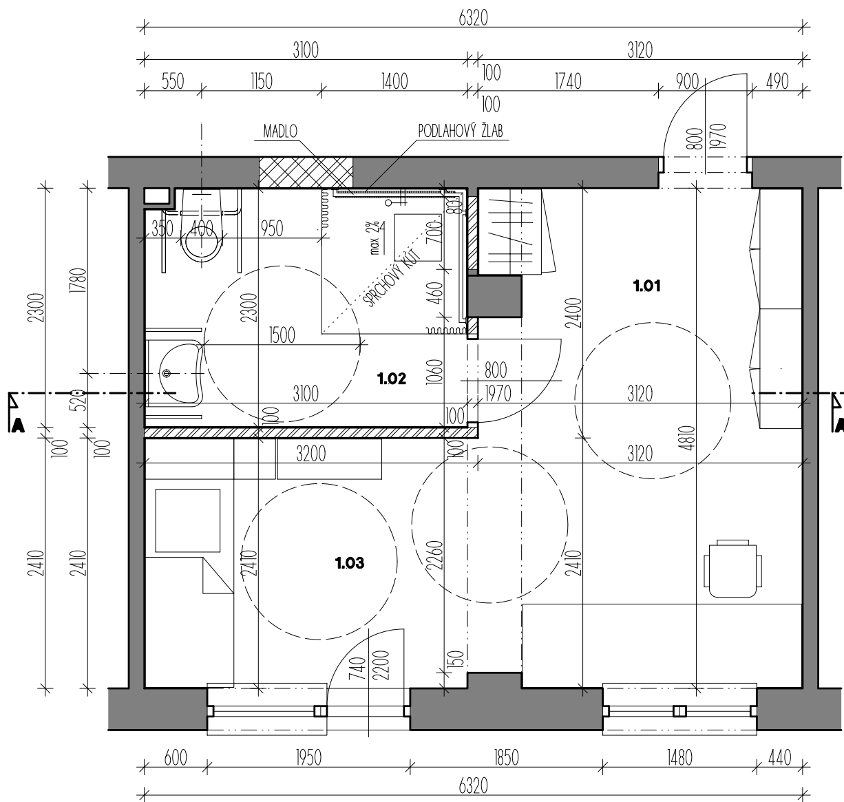
PÔDORYS IZBY - NÁVRH M 1:50
