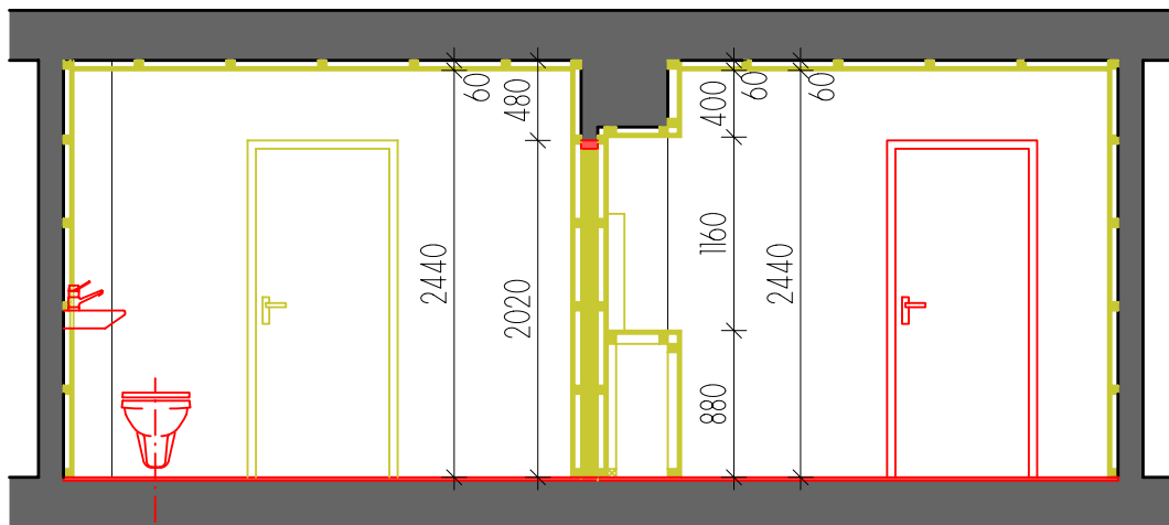
REZ A-A - BÚRACIE A MUROVACIE PRÁCE M 1:50
