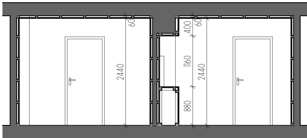
REZ A-A - SÚČASNÝ STAV M 1:50
